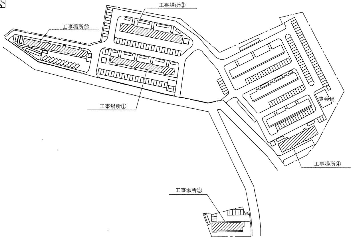
A地区配置図 S-1/2,000
