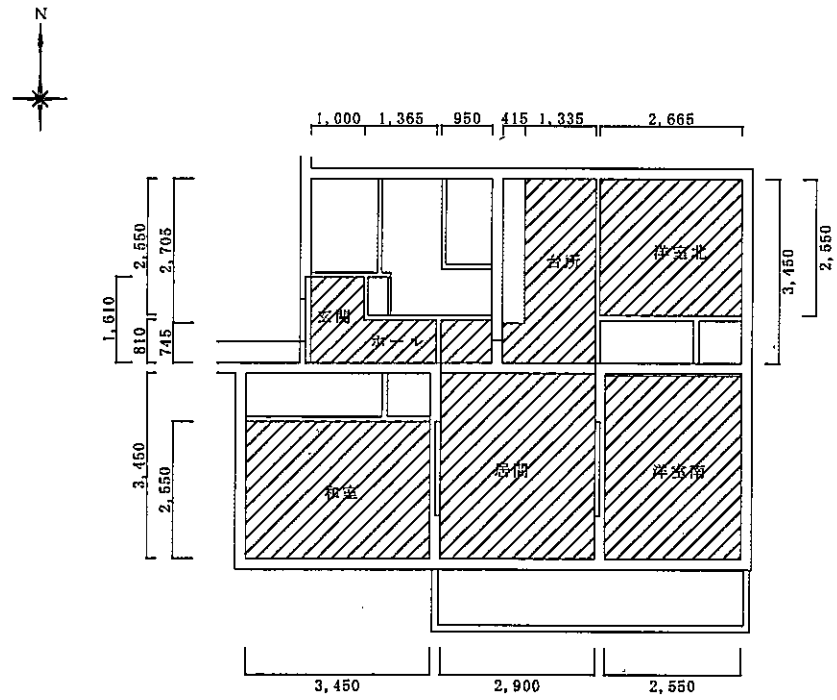
宿舎1（生野町）c規格 天井伏せ図 S=1/100
