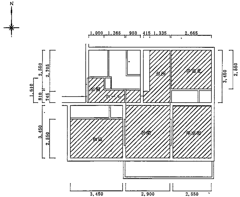
生野宿舎1棟c規格 天井伏せ図 S=1/100
