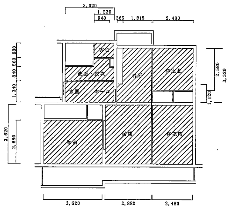
宿舎2 (生野町) c規格 天井伏せ図 S=1/100
