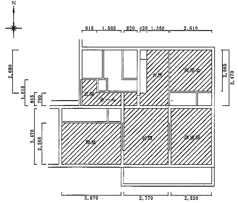
宿舎C・D (普通寺町) c規格 天井伏せ図 S=1/100
