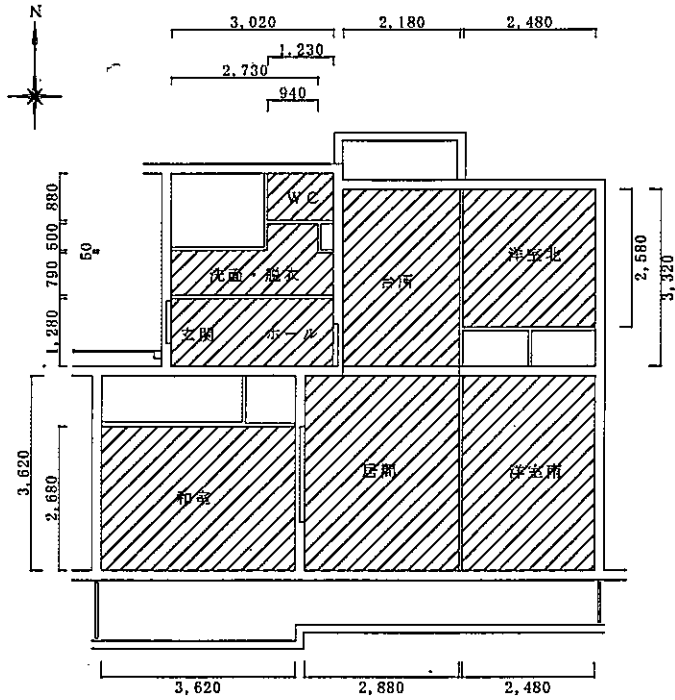
宿舎（一宮町）c規格 天井伏せ図 S=1/100
