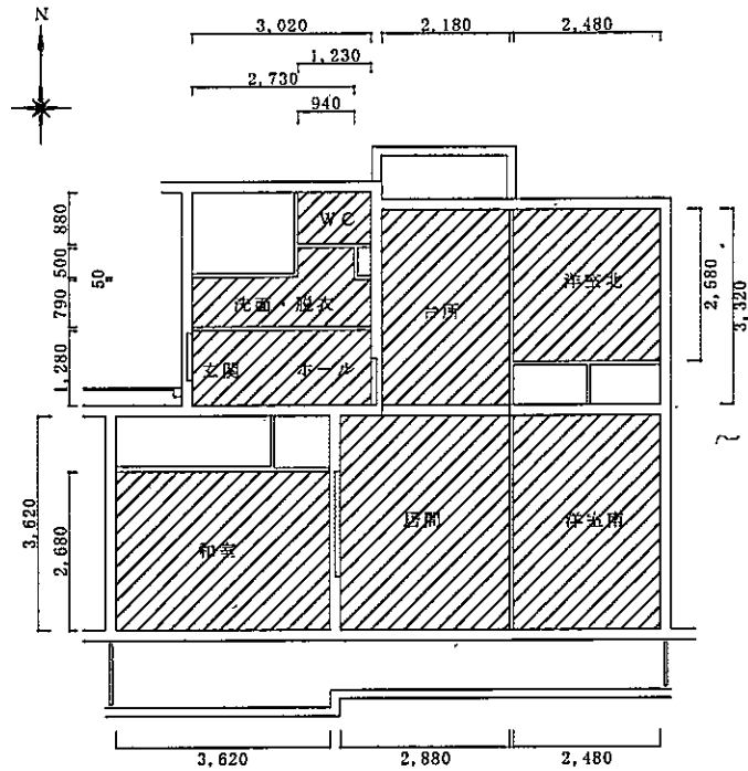
一宮宿舎c規格 天井伏せ図 S=1/100
