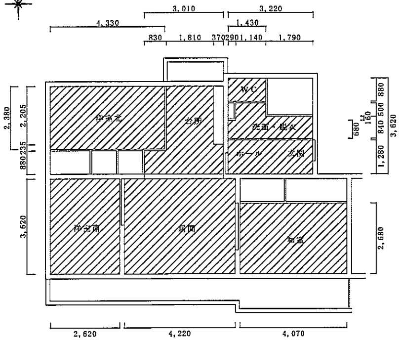
宿舎2 (生野町) d規格 天井伏せ図 S=1/100
