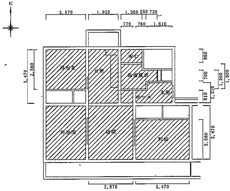
宿舎B (普通寺町) c規格 天井伏せ図 S=1/100
