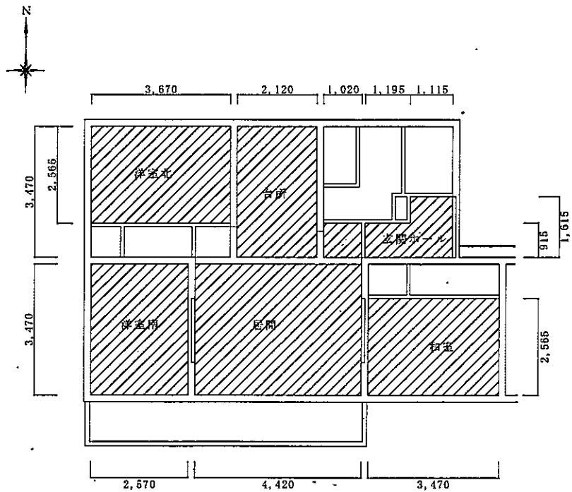
宿舎1 (生野町) d規格 天井伏せ図 S=1/100
