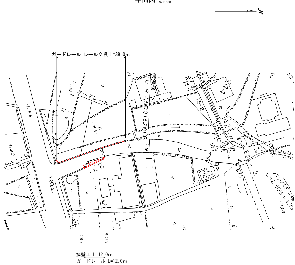
平面図 S=1:500
