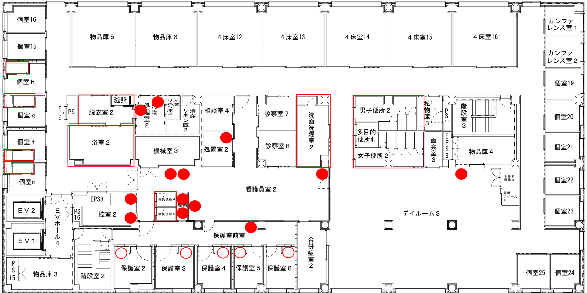
4階平面図（衛生設備配置図）
