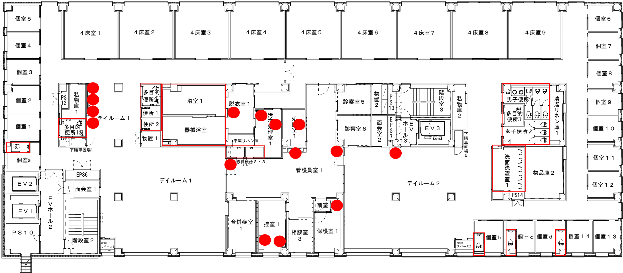
3階平面図（衛生設備配置図）
