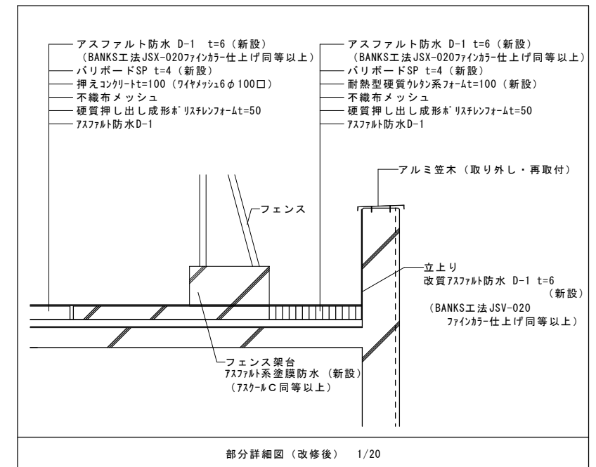
部分詳細図 (改修前) 1/20
