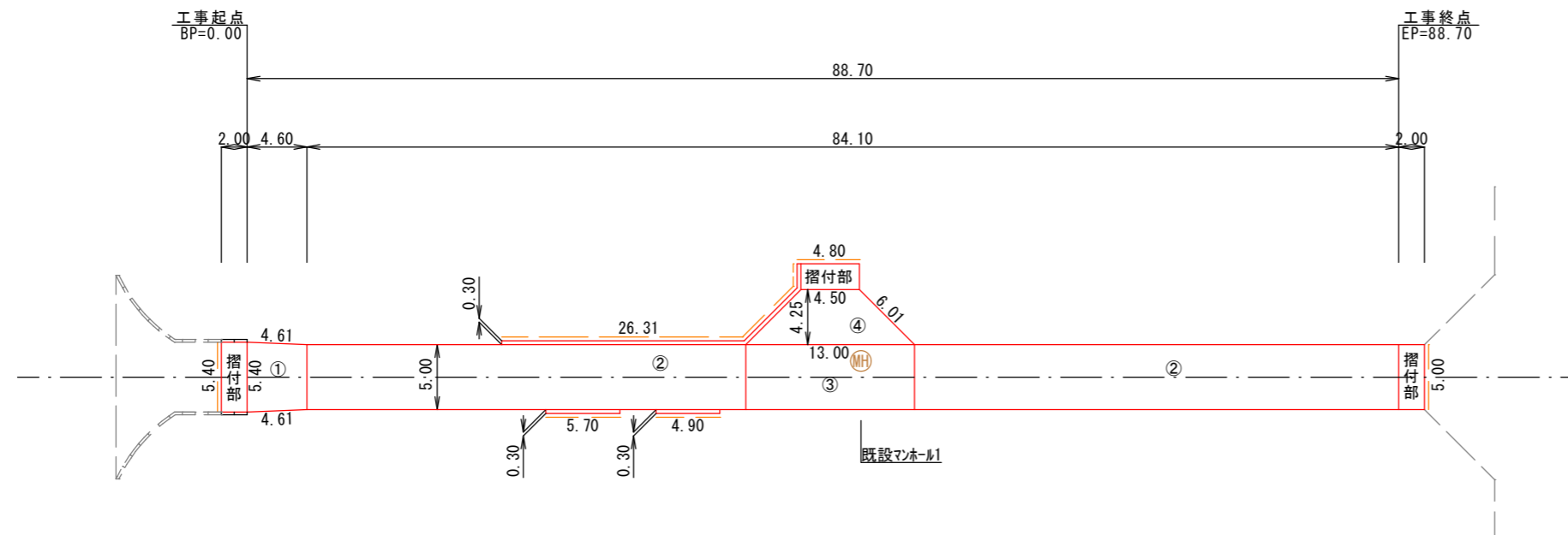
土工定規図 ①
