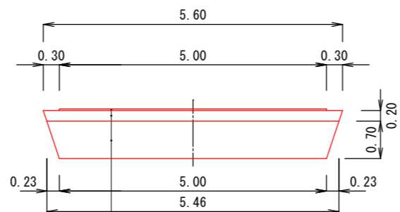
土工定規図 ②
