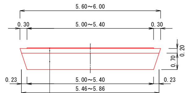
土工定規図 ①
