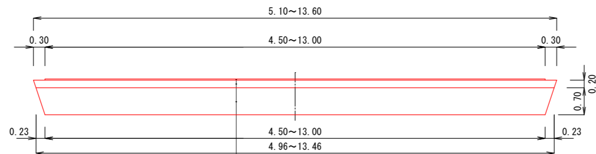
土工定規図 ④
