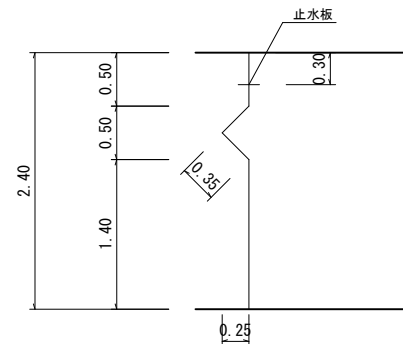
堤底
