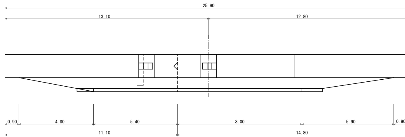
伸縮継目詳細図 S=1:50
