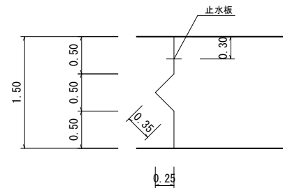
天端
