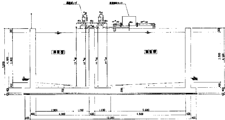
G-G 断面図 | s = 1/50
