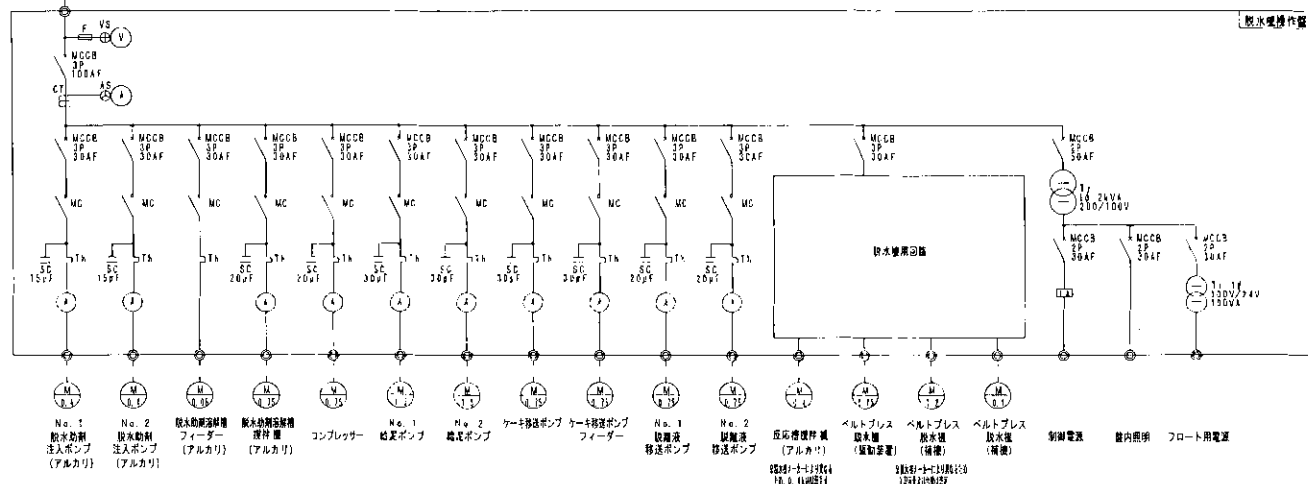
単線結線図
