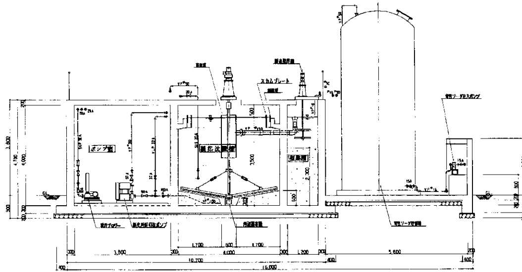
F-F 断面図 | s = 1/50
