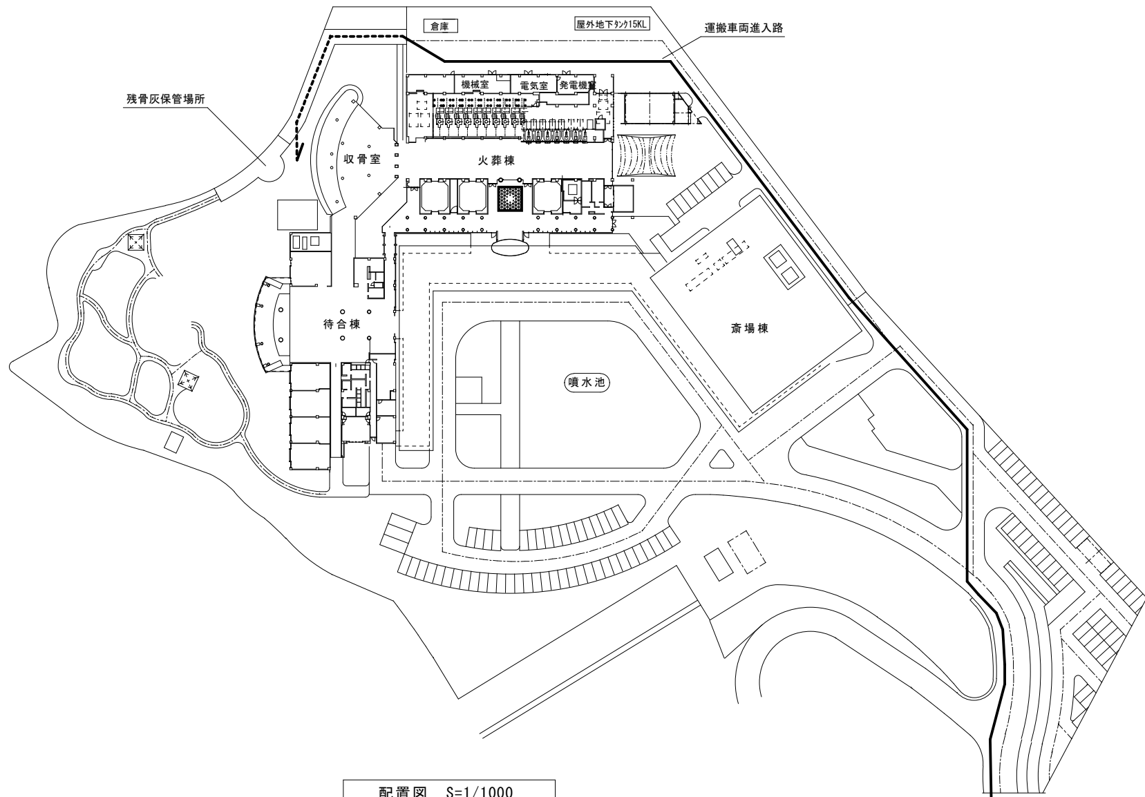
配置図 S=1/1000
