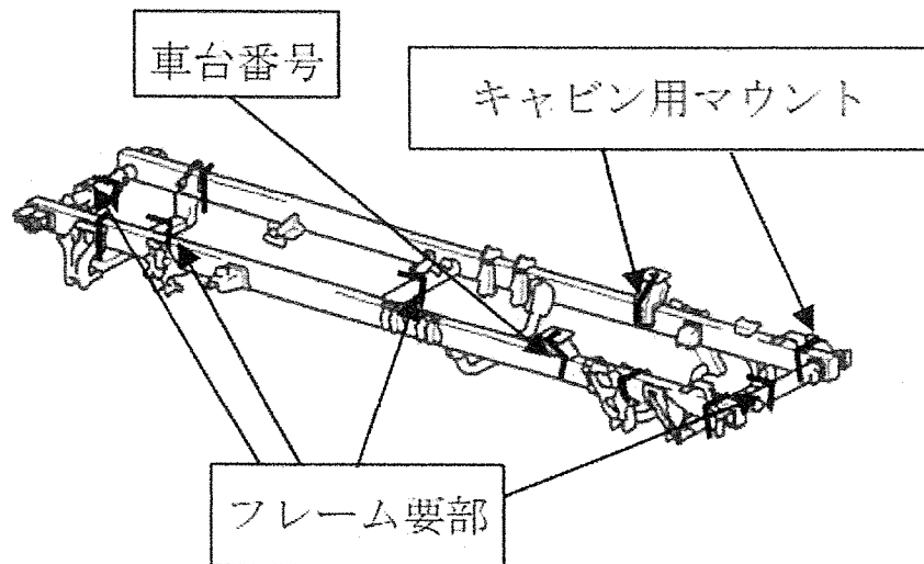
図3-高機動車外装部品及びフレームの解体・破碎図
