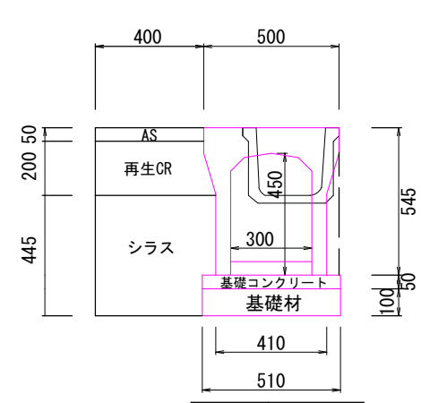
自由勾配側溝標準断面図
