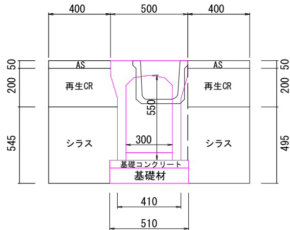
自由勾配側溝標準断面図
