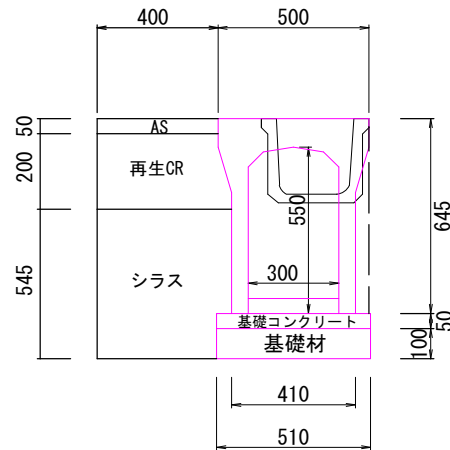
自由勾配側溝標準断面図
