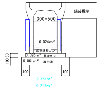
自由勾配側溝300
