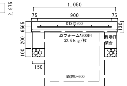
現場打蓋掛け工詳細
