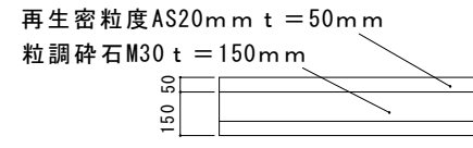
現場打蓋掛け工詳細
