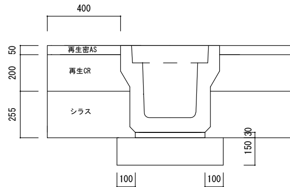
落蓋側溝300型(3種) グレーチングボルト締
