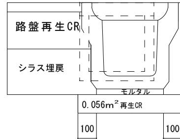
落蓋側溝300A型(消音タイプ)
