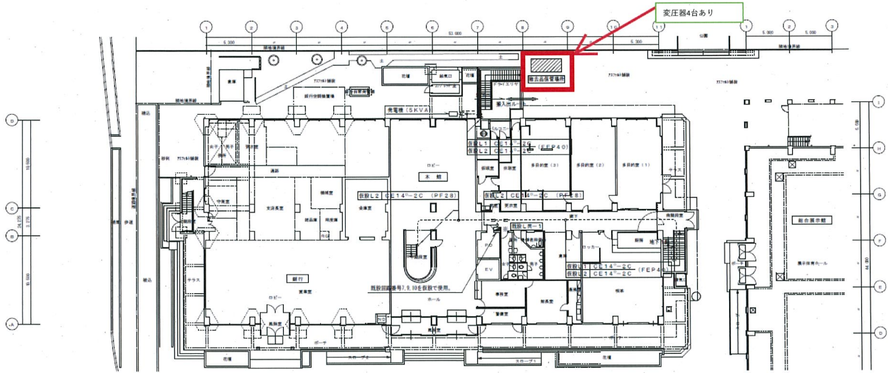
1階 平面図 1:100
