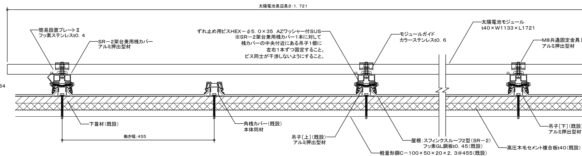
架台断面詳細図(長辺方向) S=1:5
