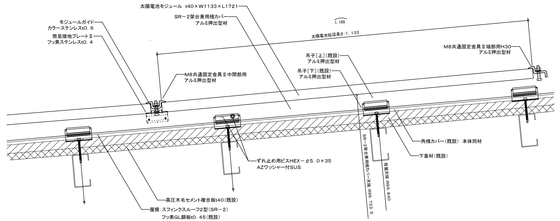
架台断面詳細図(短辺方向) S=1:5
