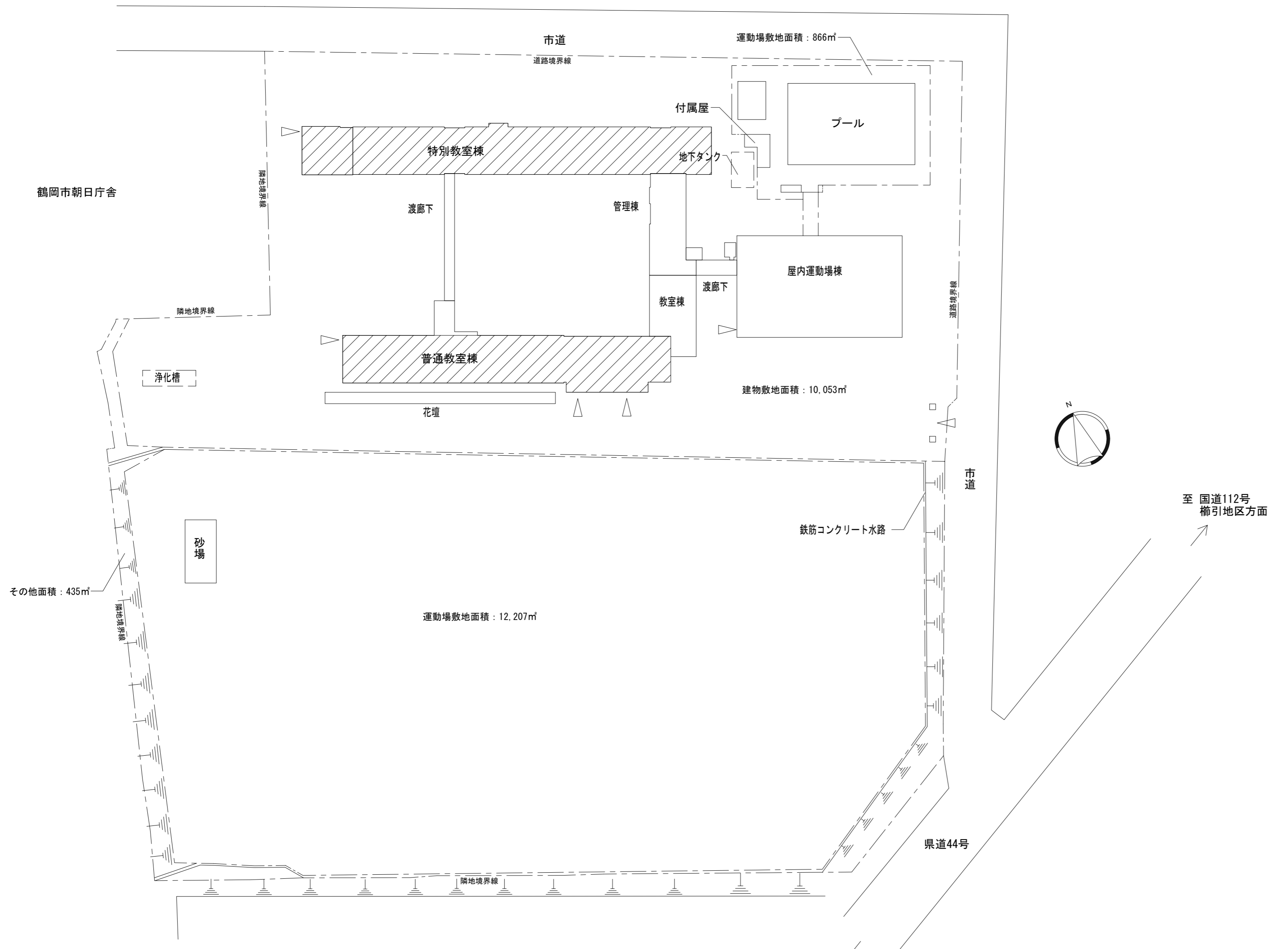
配置図 S=1/600
